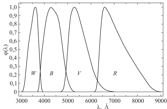
Рис. 1.4. Пример кривых реакции многоцветной фотометрической системы. Полосы фотометрической системы WBVR
