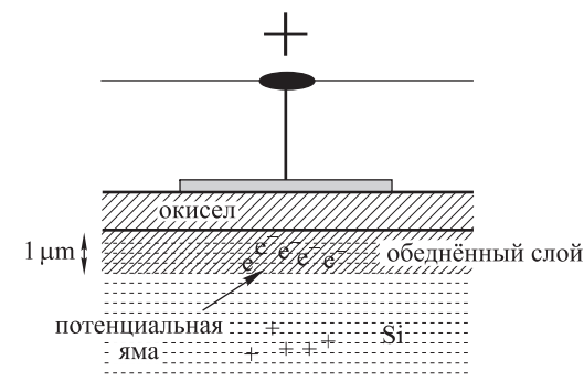
Рис. 5.1. Схема МОП-конденсатора
