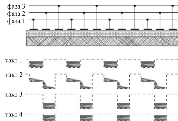
Рис. 5.2. Принцип передачи заряда между пикселями ПЗС
