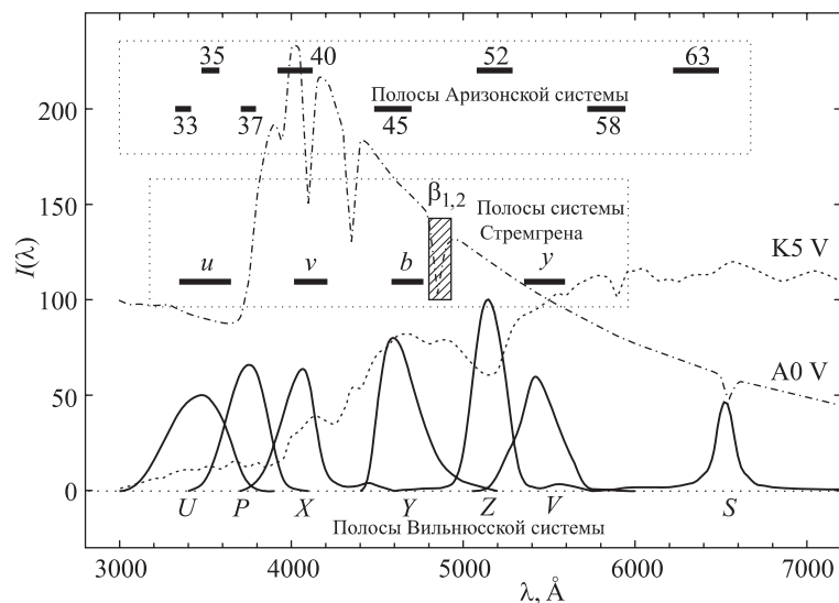
Рис. 9.7. Сравнительное положение полос системы Стрёмгrena, Аризонской и Вильнюсской среднеполосных фотометрических систем. По оси ординат даны относительные спектральные интенсивности для звёзд A0 V и K5 V
