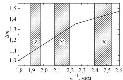
Рис. 9.5. Выбор положения полосы Y Вильнюсской системы
