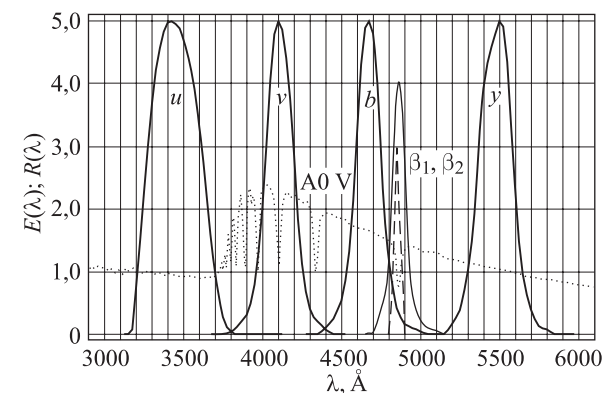
Рис. 9.1. Полосы среднеполосной системы Стрёмгрена uvby
