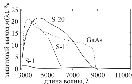
Рис. 4.6. Кривые реакции типичных фотокатодов: S20 — мультищелочной катод, S1 — серебряно-кислородно-цезиевый катод, S11 — сурьмяно-цезиевый катод, AsGa — арсенид-галлиевый катод
