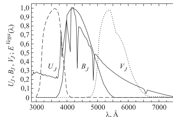
Рис. 8.1. Кривые реакции фотометрических полос системы UBV . Индекс «J» подчёркивает, что это кривые, использованные Джонсоном. Для сравнения показано распределение энергии в спектре Веги
