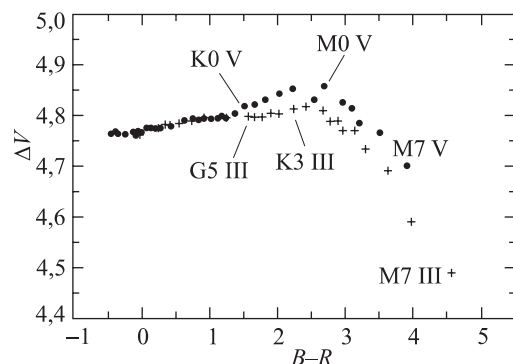
Рис. 7.7. Различие величин V для звёзд разных спектральных типов с одинаковой монохроматической величиной при \lambda 5500 Å. Кружками обозначены звёзды главной последовательности, а крестиками — гиганты
