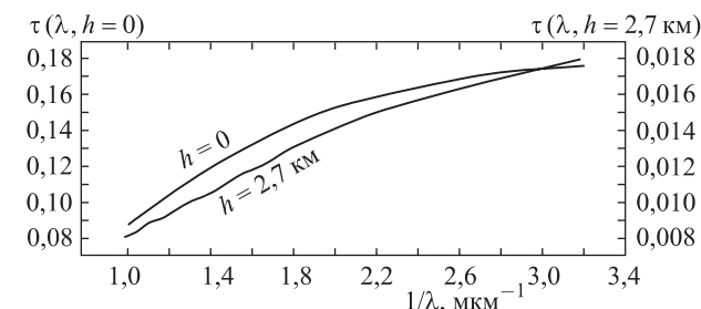
Рис. 6.8. Зависимость аэрозольной оптической толщи атмосферы от обратной длины волны
