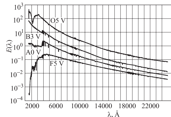
Рис. 7.3. Относительное распределение энергии в спектрах звёзд спектральных типов O5 V, B3 V, A0 V, и F5 V в спектральном диапазоне 1000–25000 Å. Масштаб по оси ординат логарифмический. Кривые сдвинуты вдоль оси ординат на произвольную константу
