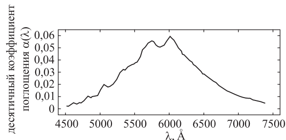
Рис. 6.11. Полосы Шаппюи поглощения озоном
