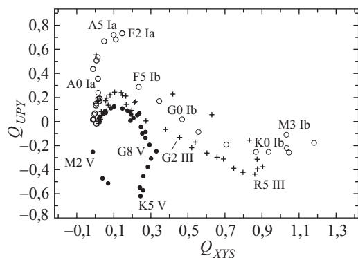
Рис. 9.10. Диаграмма Q_{UPY} , Q_{XYS} для классификации звёзд G. Обозначения как на рис. 9.8
