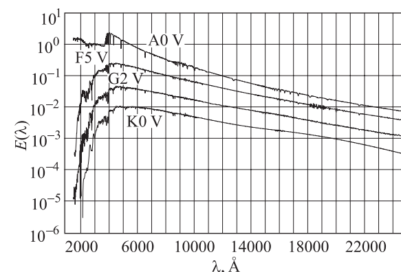
Рис. 7.5. Относительное распределение энергии в спектрах звёзд спектральных типов A0 V, F5 V, G2 V и K0 V в спектральном диапазоне 1000–25000 Å. Масштаб по оси ординат логарифмический. Кривые сдвинуты вдоль оси ординат на произвольную константу
