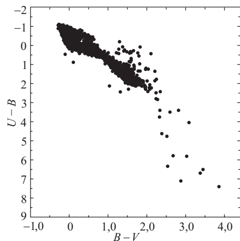
Рис. 8.2. Двухцветная диаграмма U-B , B-V для объектов Катога ярких звёзд
