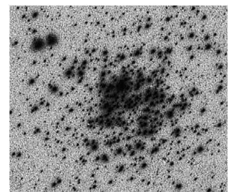
Рис. 3.3. Репродукции участка той же пластинки, что и на рис. 3.1, находящегося на расстоянии 3,3'' от центра пластинки, воспроизведённые с разным увеличением. На этом участке находится рассеянное скопление M11. На левом рисунке размер поля примерно 40' \times 40' , а на правом, увеличенном в большей степени, размер примерно 10' \times 10'
