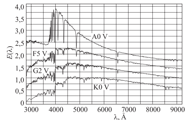
Рис. 7.6. Относительное распределение энергии в спектрах звёзд A0 V, F5 V, G2 V и K0 V в спектральном участке, соответствующем оптическому окну прозрачности атмосферы. Кривые сдвинуты вдоль оси ординат на произвольную константу
