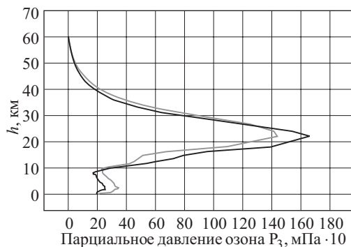
Рис. 6.9. Типичное распределение количества атмосферного озона с высотой над уровнем моря в северном полушарии для зимнего и летнего сезонов
