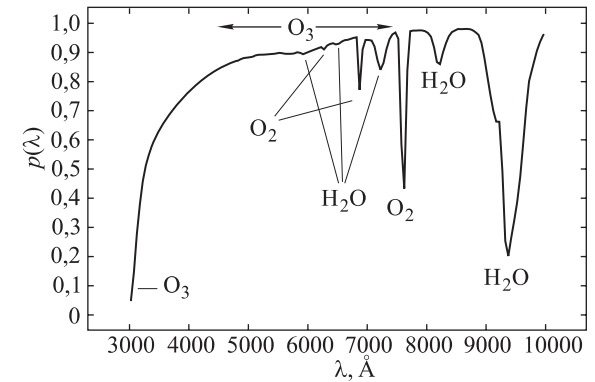
Рис. 6.16. Сводная зависимость прозрачности чистой атмосферы от длины волны
