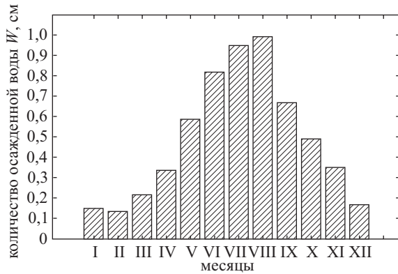
Рис. 6.13. Годовой ход количества осаджённой воды в Тянь-Шаньской высокогорной астрономической обсерватории (высота 2760 м)
