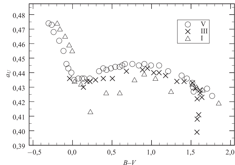
Рис. 11.3. Зависимость коэффициента атмосферной экстинкции a_U в полосе U системы UBV от показателя цвета B-V для звёзд различных спектральных типов. Расчет выполнен для высокогорной обсерватории
