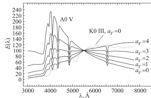
Рис. 7.16. Изменение наблюдаемого распределения энергии в спектре звезды A0 под воздействием межзвёздного поглощения света. Для сравнения приведена кривая для непокрашенённой звезды K0 III
