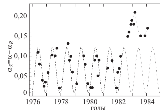
Рис. 6.6. Циклический характер изменения аэрозольной экстинкции в Заилийском Алатау. По данным В.Г. Мошкалева, полученным в высокогорной обсерватории близ Алма-Аты
