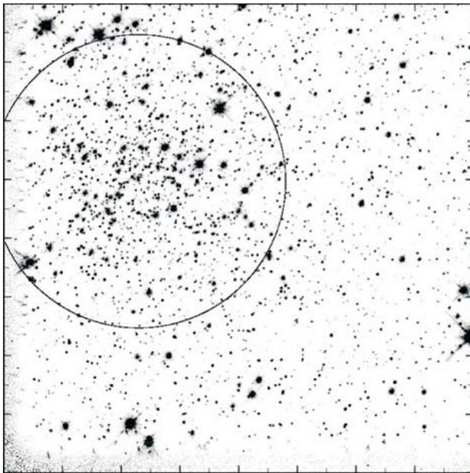
Рис. 5.9. ПЗС-фрейм ядра шарового скопления NGC6752, полученного на HST изображений) общей функцией рассеяния, варьируя только амплитуду максимумов, то логарифмы этих амплитуд будут пропорциональны логарифмам потоков излучения от измеряемых звёзд.
