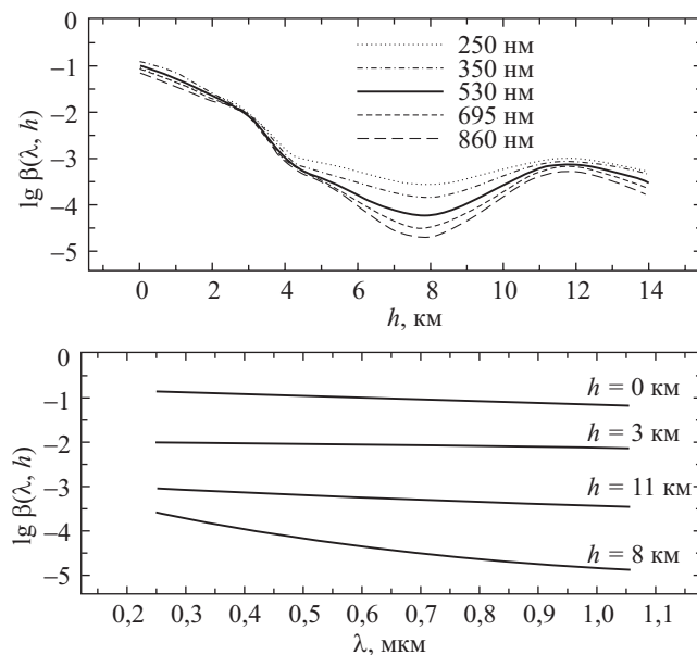
Рис. 6.7. На верхней панели — зависимость \beta_\lambda от высоты над уровнем моря для пяти длин волн. Видно, что в районе тропопавзы аэрозольный коэффициент ослабления света имеет инверсный характер. На нижней панели — зависимость \beta_\lambda от длины волны на четырёх уровнях. Видно, что на высоте 8 км над уровнем моря наклон зависимости наиболее крутой. Это свидетельствует о том, что самые мелкие аэрозольные частицы находятся под тропопавзой
