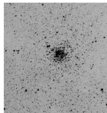
Рис. 3.3. Репродукции участка той же пластинки, что и на рис. 3.1, находящегося на расстоянии 3,3'' от центра пластинки, воспроизведённые с разным увеличением. На этом участке находится рассеянное скопление M11. На левом рисунке размер поля примерно 40' \times 40' , а на правом, увеличенном в большей степени, размер примерно 10' \times 10'
