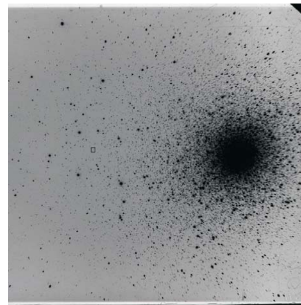
Рис. 3.10. Репродукция части пластинки, полученной на 5-метровом паломарском рефлекторе. Область шарового скопления М5. Центр оригинального негатива показан прямоугольником
