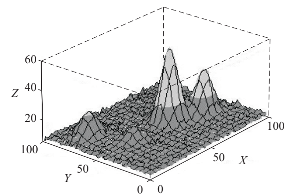
Рис. 5.6. Трёхмерные изображения четырёх звёзд из PSF-фрейма
