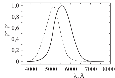
Рис. 1.2. Дневная (сплошная линия) и ночная (штриховая линия) кривые спектральной чувствительности человеческого глаза
