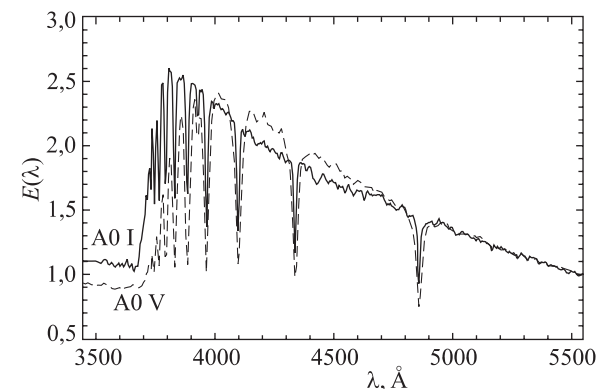
Рис. 7.11. Распределение энергии в спектрах звёзд класса A0 разных классов светимости
