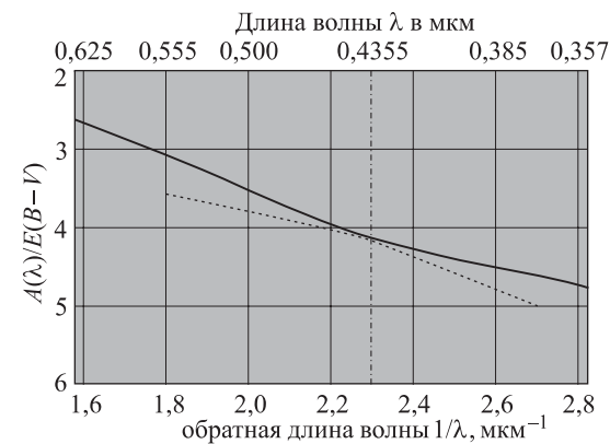
Рис. 7.14. Нормальный закон Уитфорда межзвёздного поглощения света. Светлые пунктирные линии экстраполируют отрезки линии нормального закона по обе стороны от точки излома, показывая отклонения от закона \lambda^{-1}
