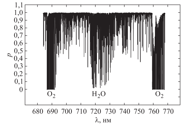
Рис. 6.14. Полосы поглощения молекулярного кислорода в области фотометрических полос V и R . Между полосами кислорода расположена полоса поглощения водяного пара
