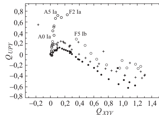
Рис. 9.9. Диаграмма Q_{UPY} , Q_{XYV} для классификации звёзд А–F. Обозначения как на рис. 9.8
