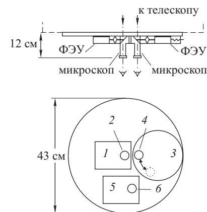
Рис. 4.8. Простейший трёхканальный фотометр Репсаке, изготовленный в Вильнюсе и используемый для исследования микроколебаний блеска белых карликов: 1 — блок канала первой звезды; 2, 4, 6 — микроскопы; 3 — подвижный блок канала второй звезды; 5 — блок канала фона
